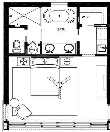
CABANA
